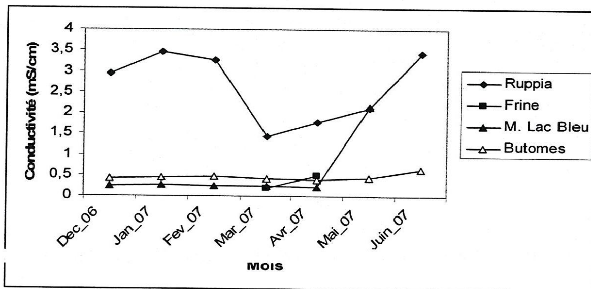
Fig. 11. Variation mensuelle de la conductivité dans les mares de la Numidie orientale.
