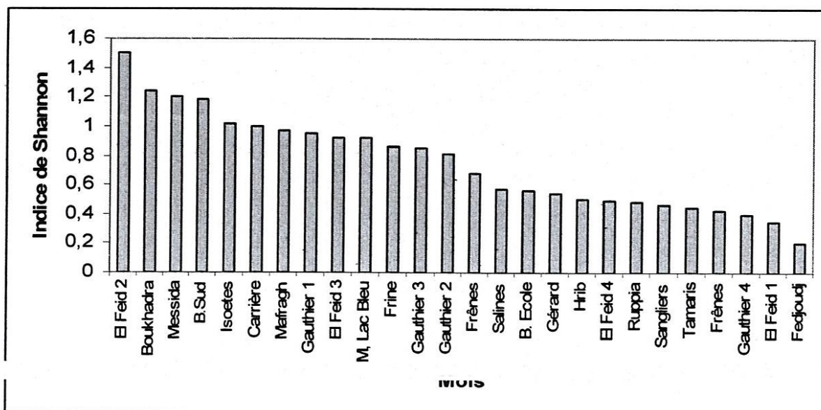
Fig. 36. Variation de l'indice de diversité de Shannon entre les mares de la Numidie orientale.
