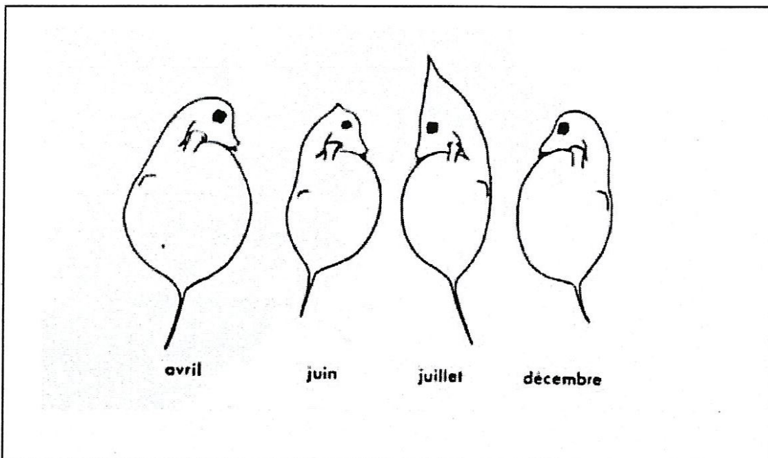
Fig. 5. Exemple de cyclomorphose : Daphnia galeata dans la Mindelsee (Einsel, 1966).
