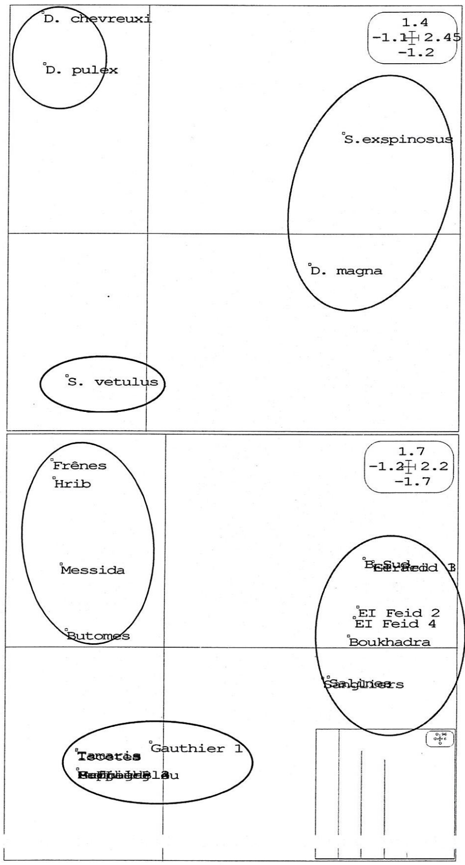
Fig. 40. Axe 1x2. Analyse factorielle des correspondances (AFC), (05 Taxa et 26 mares).
