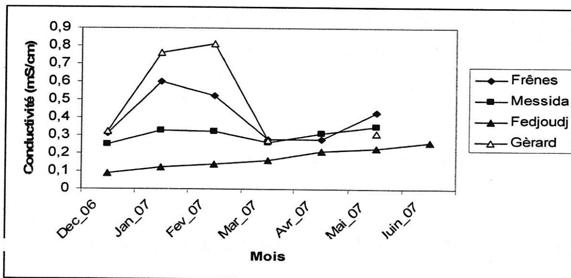
Fig. 10. Variation mensuelle de la conductivité dans les mares de la Numidie orientale.
