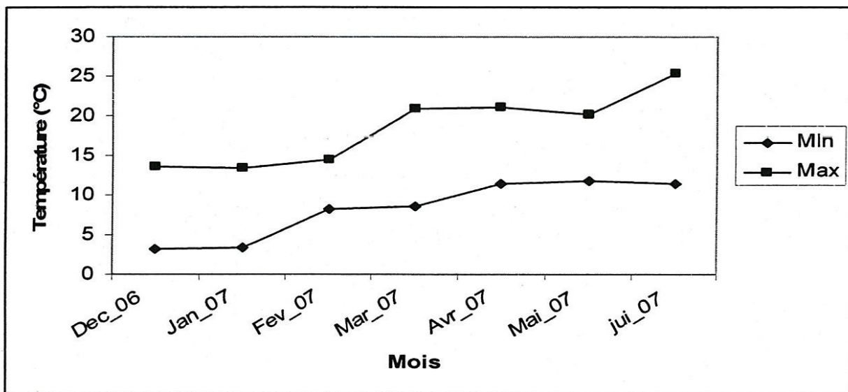
Fig. 15. Variation mensuelle de la température dans les mares de la Numidie orientale.
