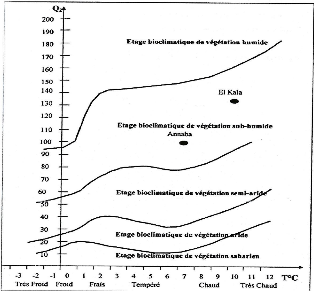
Fig.7. Situation des stations météorologiques de référence pour le climat de la Numidie dans le climagramme d'Emberger.
