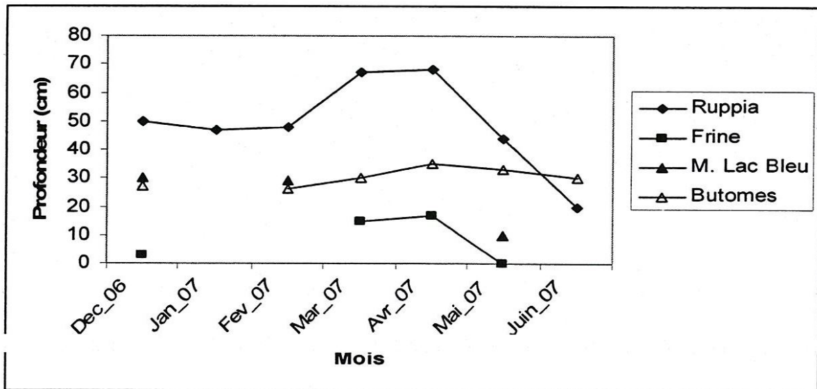
Fig. 13. Variation mensuelle de la profondeur de l'eau à travers les mares de la Numidie orientale.
