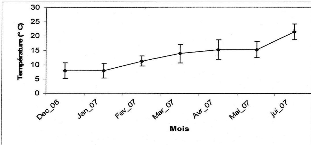
Fig. 14. Variation mensuelle moyenne de la température dans les mares de la Numidie orientale.
