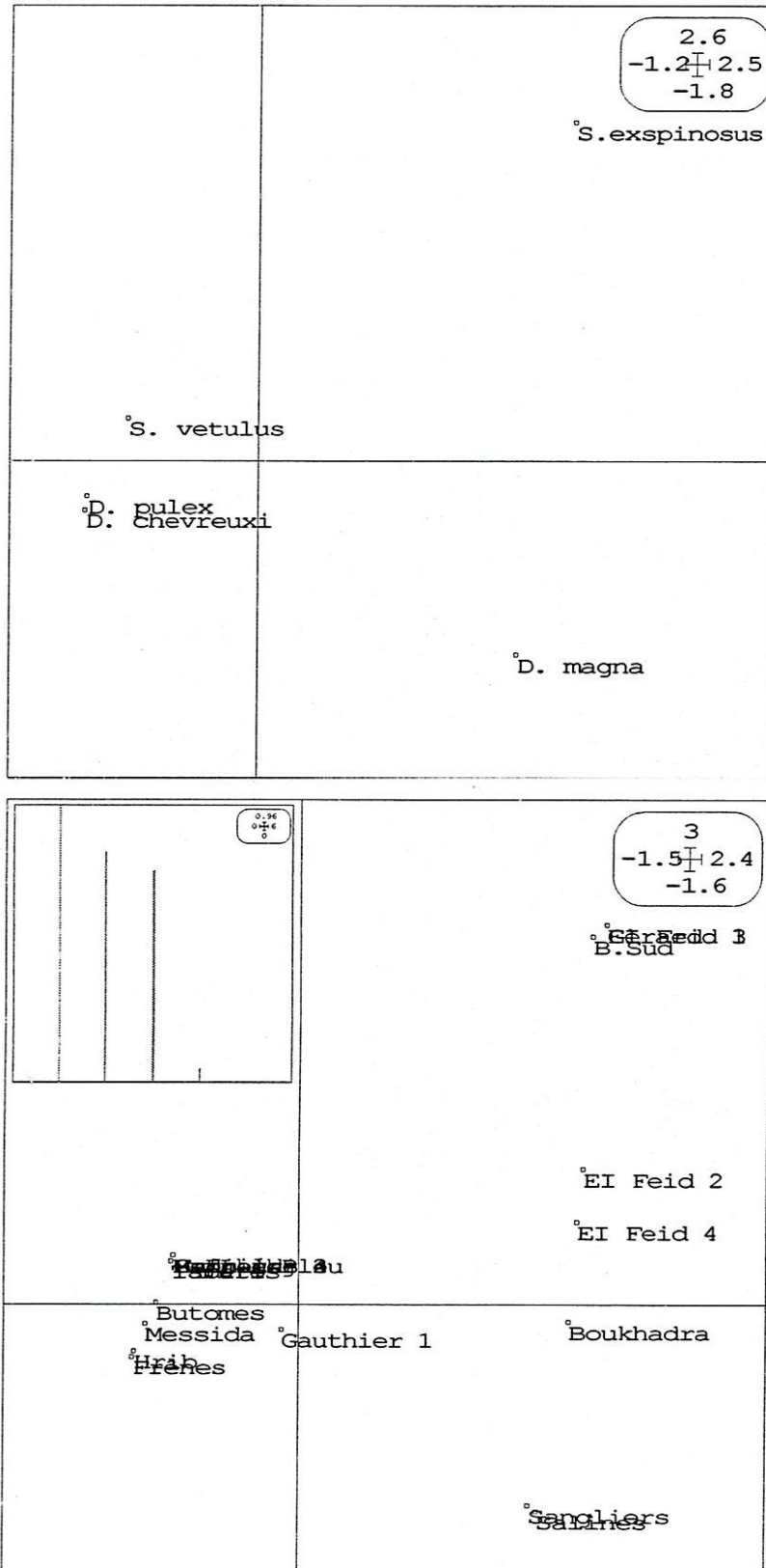
Fig. 41. Axe 1x3. Analyse factorielle des correspondances (AFC), (05 Taxa et 26 mares).
