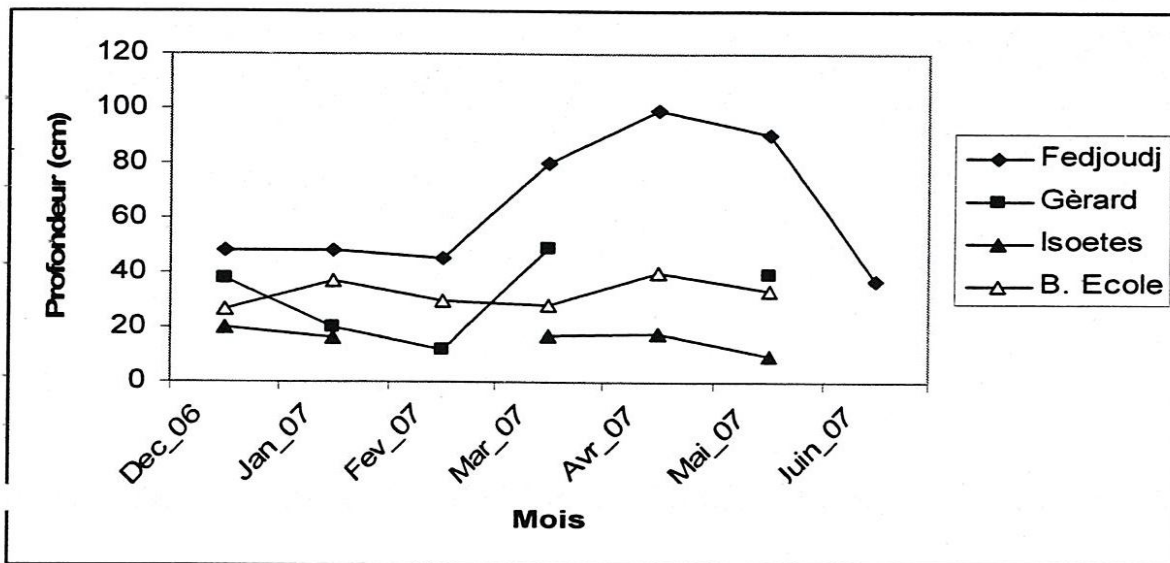
Fig. 12. Variation mensuelle de la profondeur de l'eau à travers les mares de la Numidie orientale.
