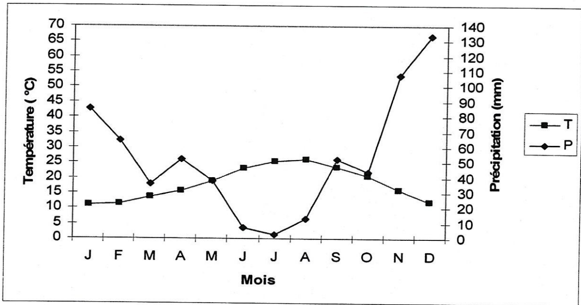
Fig.8. Diagramme ombro-thermique de la région d'El Kala.
