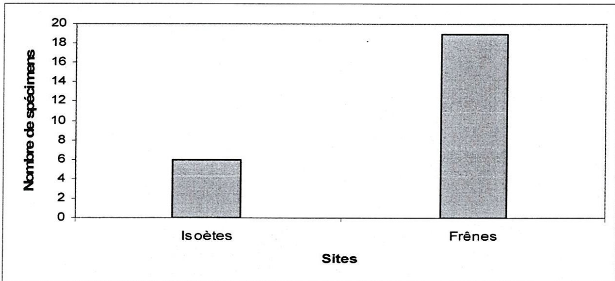
Fig. 20. Abondance des populations de Daphnia pulex dans les mares de la Numidie orientale.
