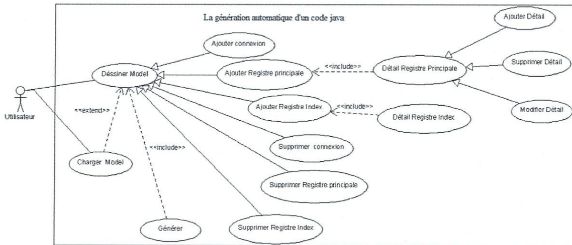
Figure 4.2 : Diagramme de cas d'utilisation.
