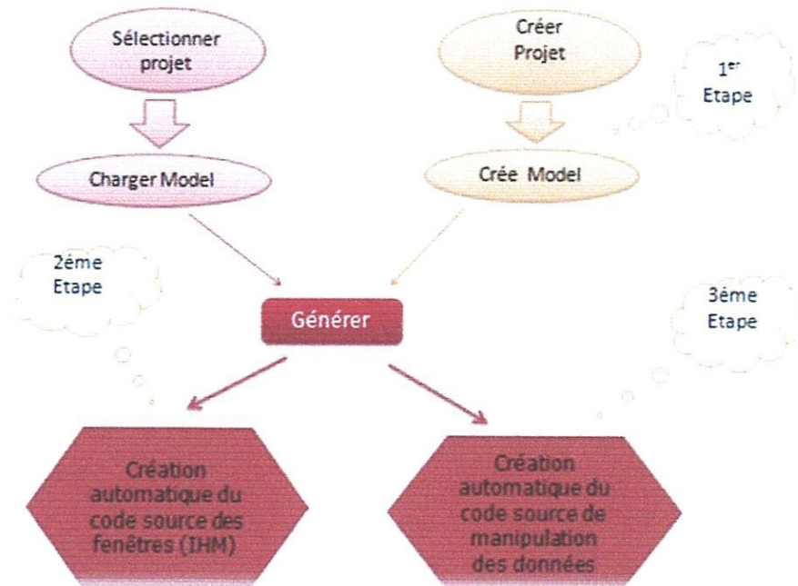
Figure 4.1 : Représentation de notre travail
