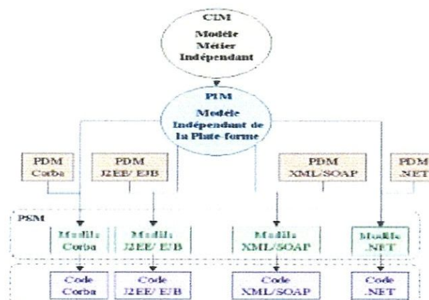
Figure 2.2 : Utilisation des modèles pour réaliser une application. [11]
