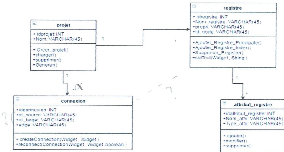
Figure 4.3 : Diagramme de classes.
