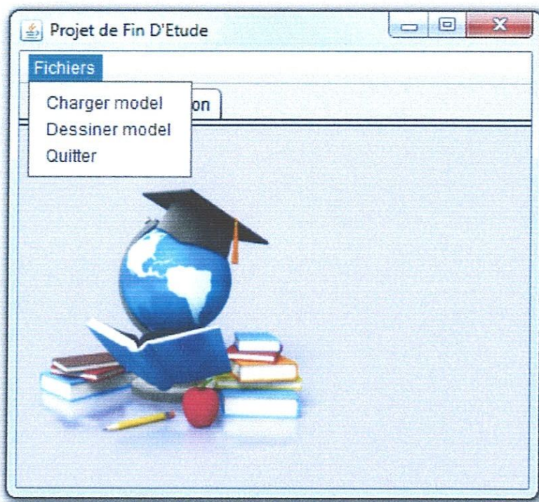
Figure 5.1 : Interface d'accueil
