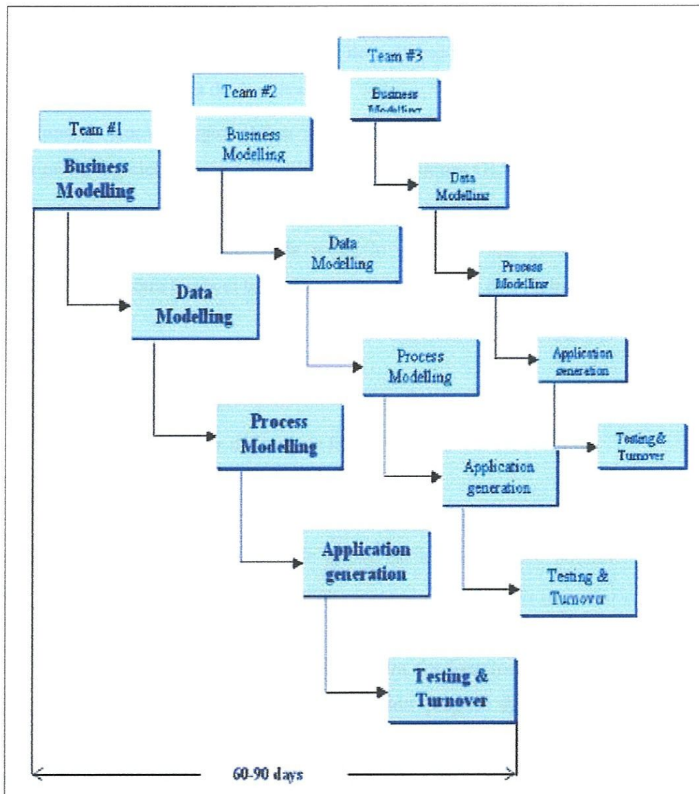
Figure 3.1 : RAD modèle
