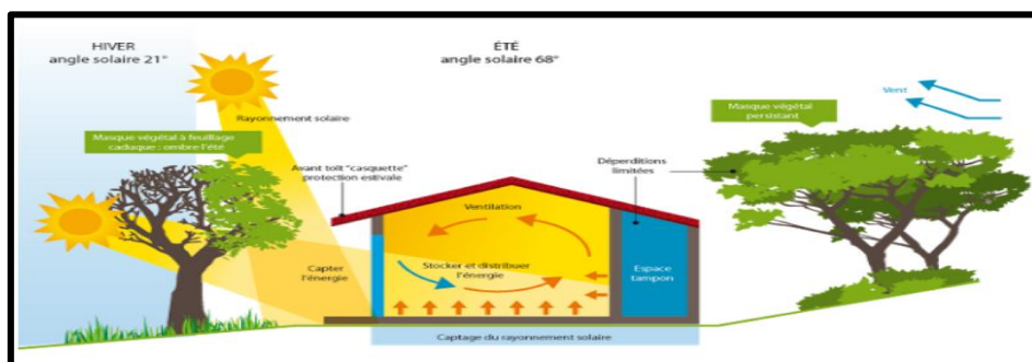
Figure 17 : principes de base d'une conception bioclimatique (implantation et organisation spatiale) (source : e-rt2012, 2017).
