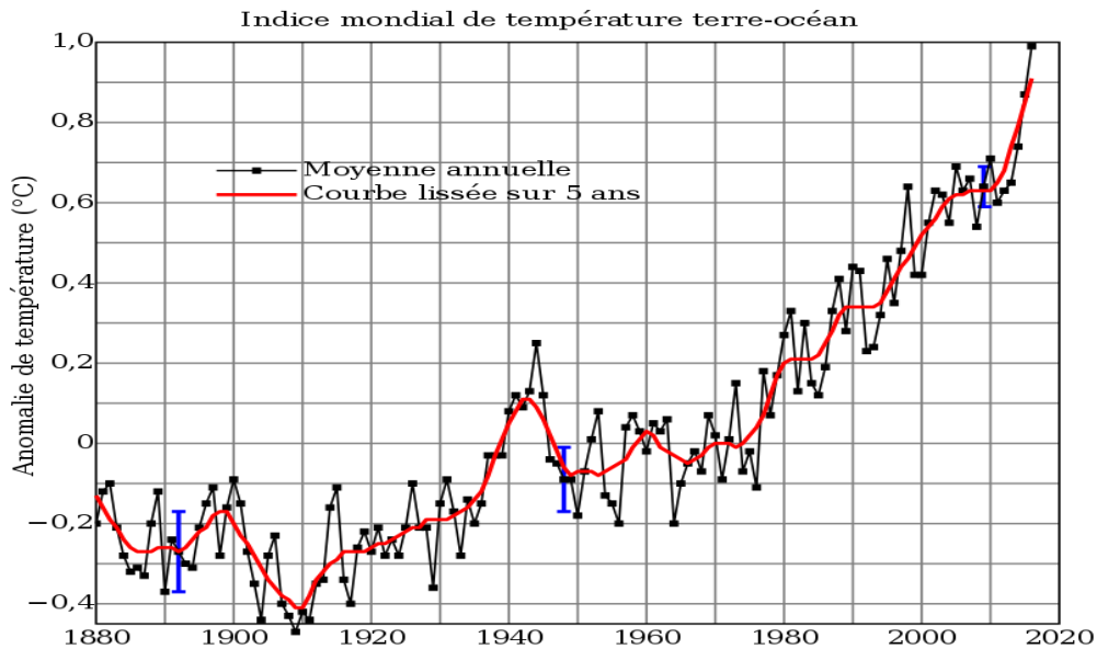
Figure 2 : Graphique des anomalies des températures globales moyennes de surface par rapport à la moyenne 1951-1980. (Source: NASA Goddard Institute for Space Studies)
