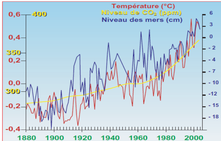
Figure 3 : évaluation des variations de température et de niveau des mers autour des niveaux moyens, évolutions des rejets de CO 2 . (Source: NASA, SHOM, CNRS.)
