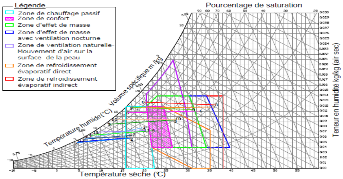
Figure 61: Diagramme psychrométrique de Guelma (Source: Auteur).
