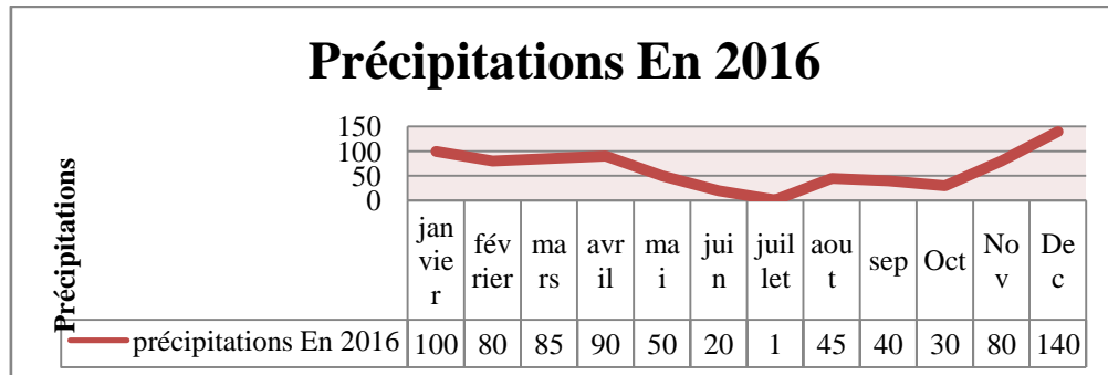
Figure 56 : variation des précipitation mensuelles (période 2016) (source : auteur)..
