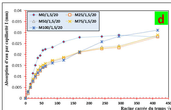
Figure IV-17 Cinétique d'absorption d'eau par capillarité en fonction de a) taux de substitution de SD par SR de mortier témoin, b) avec 0.5% de PET-F 20 mm, c) avec 1% de PET-F 20 mm, d) avec 1.5% de PET-F 20 mm et e) de 2% de PET-F 20 mm.
