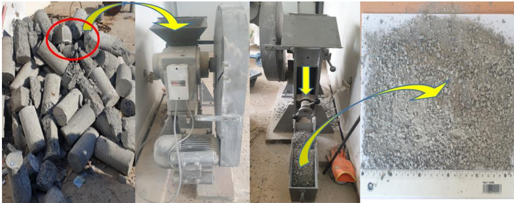
Figure III-2 : Sable recyclé
