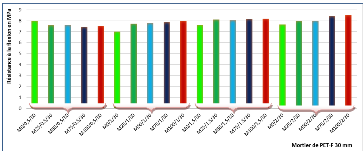
Figure IV-9 R f des mortiers en fonction du taux de PET-F 30 mm.
