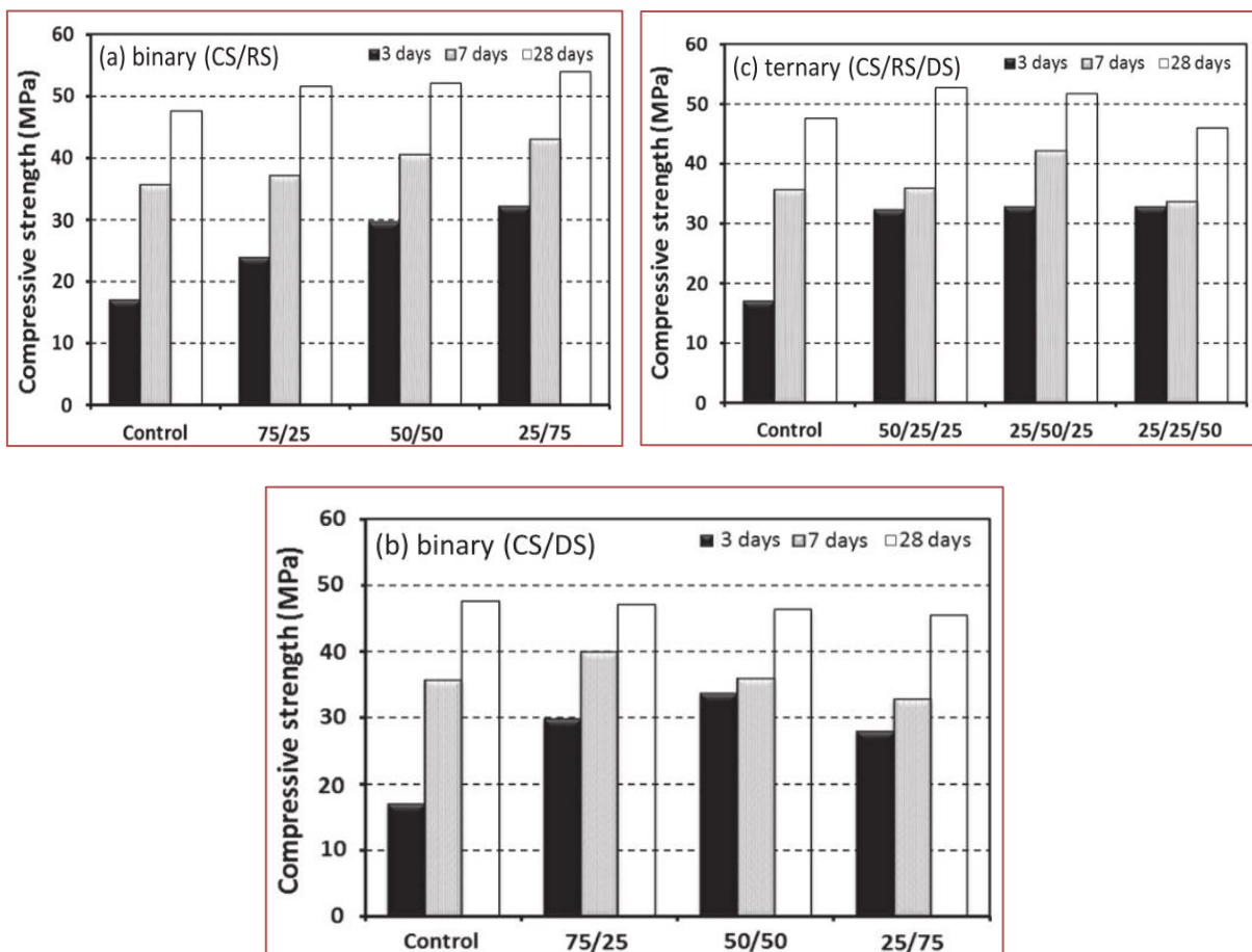
Figure I-15 Rc à (3, 7 et 28 jours) d'un mortier composé de : (a)sable binaire (CS/RS), (b)sable binaire (CS/DS), et (c)sable ternaire (CS /RS/DS).
