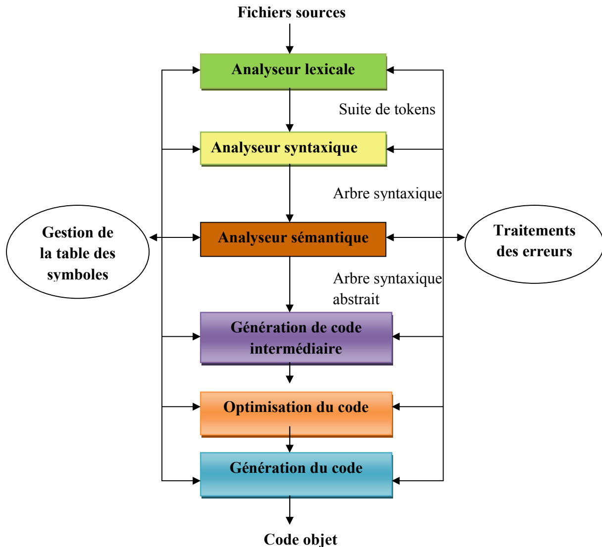
Figure 2.2-Structure d'un compilateur.
