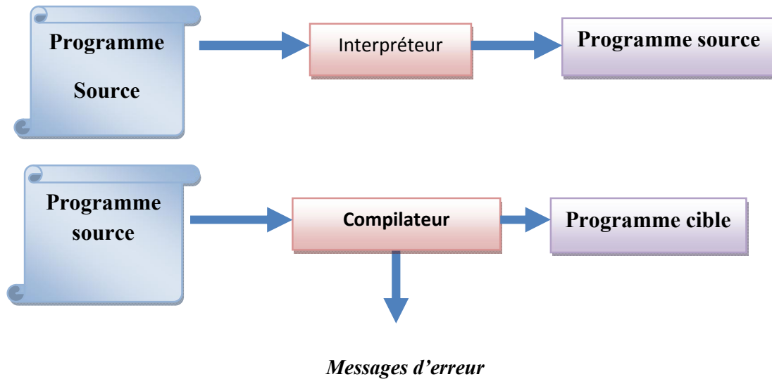
Figure2.1-Compilateur.
