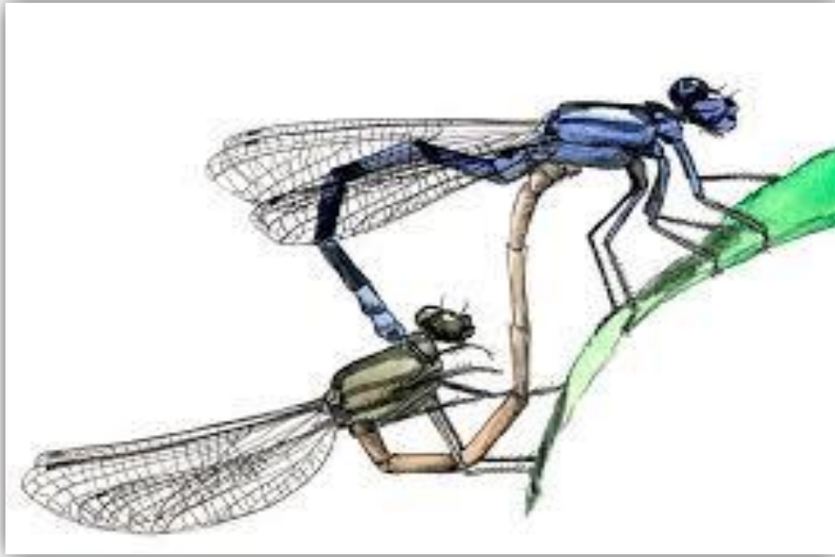
Figure 13: La copulation chez les odonates.
