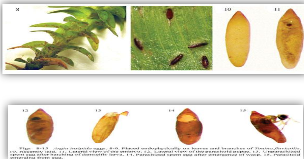
Figure 10 : Les œufs de type de ponte endophytique.
